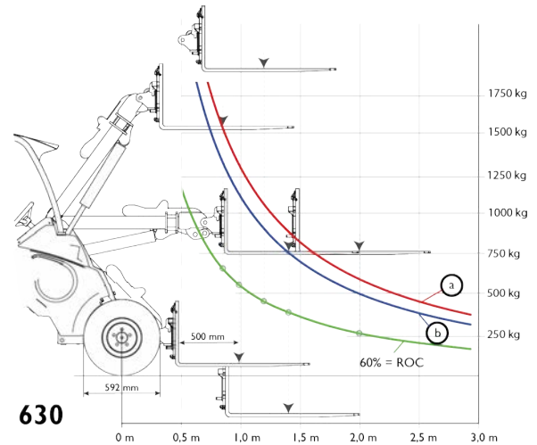
Diagramme de charge 630/635/640
